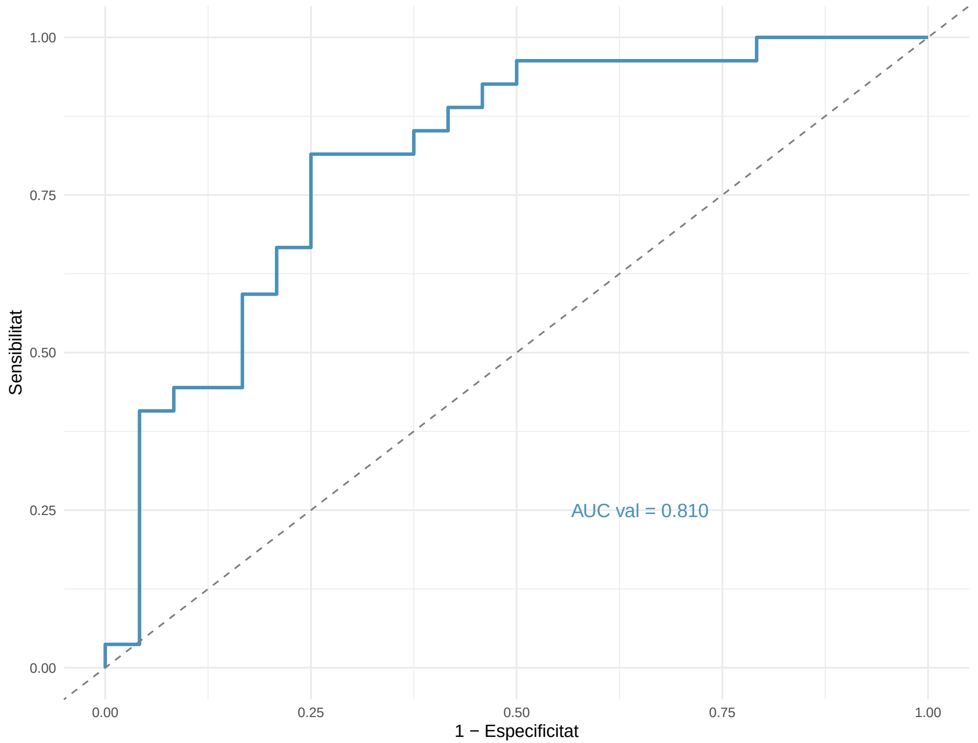
Corba ROC — SVM-RBF (val)
